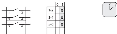
2.423 Прекъсвач 0-1 (3 - полюсен)
