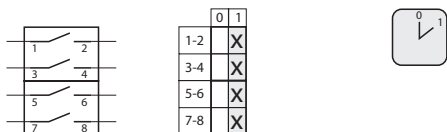
3.8220 Прекъсвач 0-1 (5 - biegunowy)
