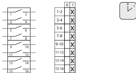
5.8220 Прекъсвач 0-1 (9 - полюсен)
