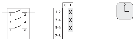
2.4226 Прекъсвач 0-1 (4 - полюсен)
