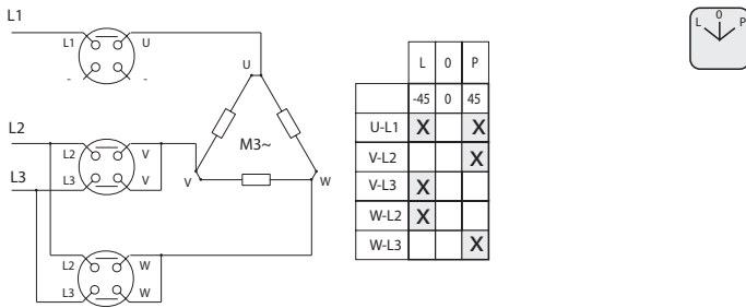
4.883 Превключвател за измерване на напрежение
