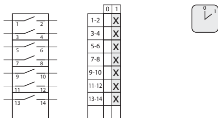
4.824 Прекъсвач 0-1 (8 - полюсен)
