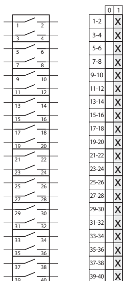
10.821 Trennschalter 0-1 (20-polig)
