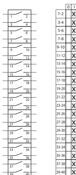
10.821 Переключатель 0-1 (20 - полюсный)
