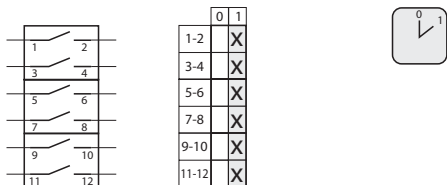
3.8210 Переключатель 0-1 (6 - полюсный)
