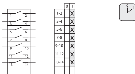
4.824 Переключатель 0-1 (8 - полюсный)
