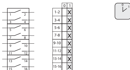
5.8220 Переключатель 0-1 (9 - полюсный)
