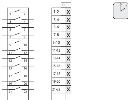
6.8210 Переключатель 0-1 (11 - полюсный)
