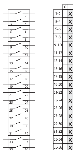
9.821 Переключатель 0-1 (18 - полюсный)
