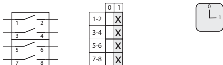
2.8210 Переключатель 0-1 (4 - полюсный)
