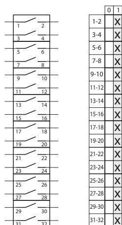
9.8210 Переключатель 0-1 (17 - полюсный)
