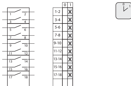
5.822 Переключатель 0-1 (10 - полюсный)
