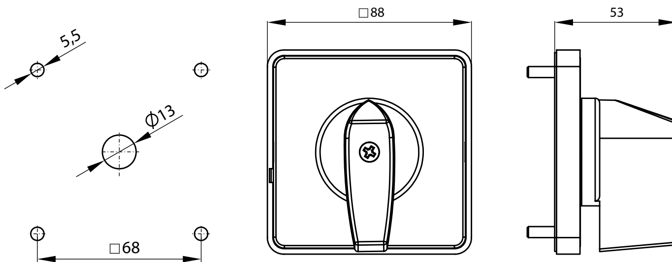
Rozměrový náčrt 68 mm×68 mm (4 šrouby M5×20)
