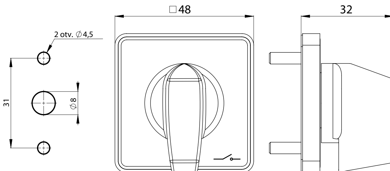
Rozměrový nákres 31 mm (2 šrouby M4x14)
